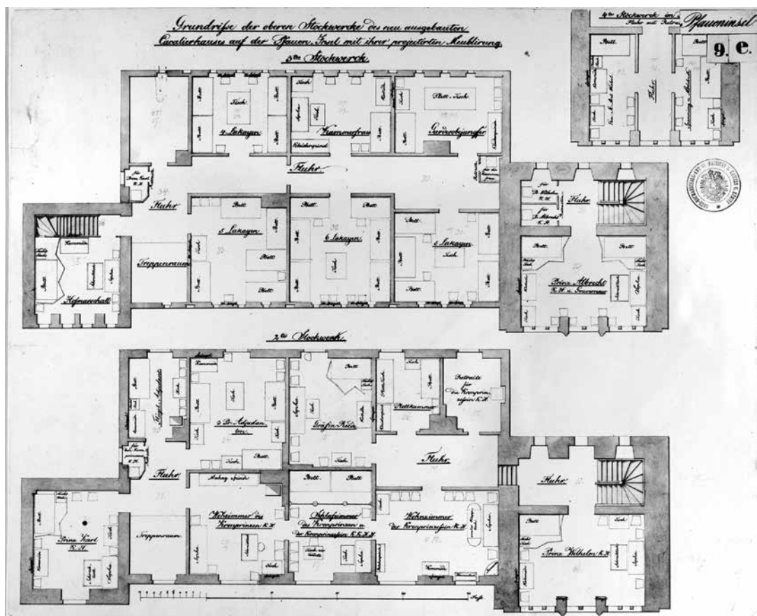
Il. 12. Rysunek rzutów kondygnacji Kavalierhaus z naniesionym układem umeblowania wnętrza, 1824 r., niesygnowany. Fotokopia w zbiorach ISPAN, sygn. dep. ZMOiZ, nr 1307
