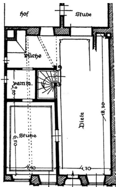
Il. 4. Rzuty parteru i pierwszego piętra kamienicy cechu kramarzy w Elblągu, wg Rendschmidt, Das alte Elbinger Bürgerhaus... , il. 49
