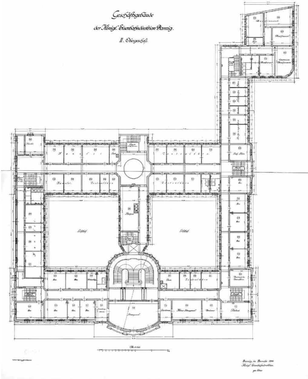
II. 4. Gmach Dyrekcji Kolei w Gdańsku, rzut II piętra, Technische Universität Berlin, Architekturmuseum in der Universitätsbibliothek, Inv.-Nr. 30803
